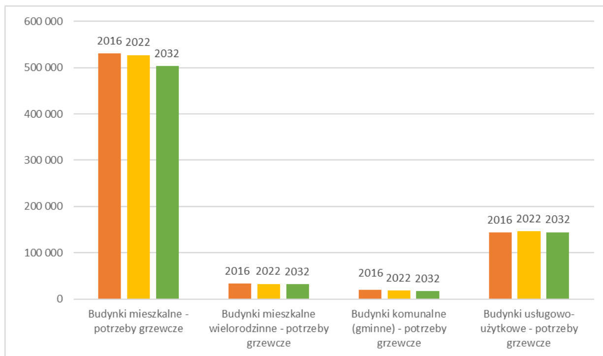
Wykres 8. Zużycie energii dla budownictwa na terenie gminy łącznie na potrzeby grzewcze wg scenariusza optymalnego.
