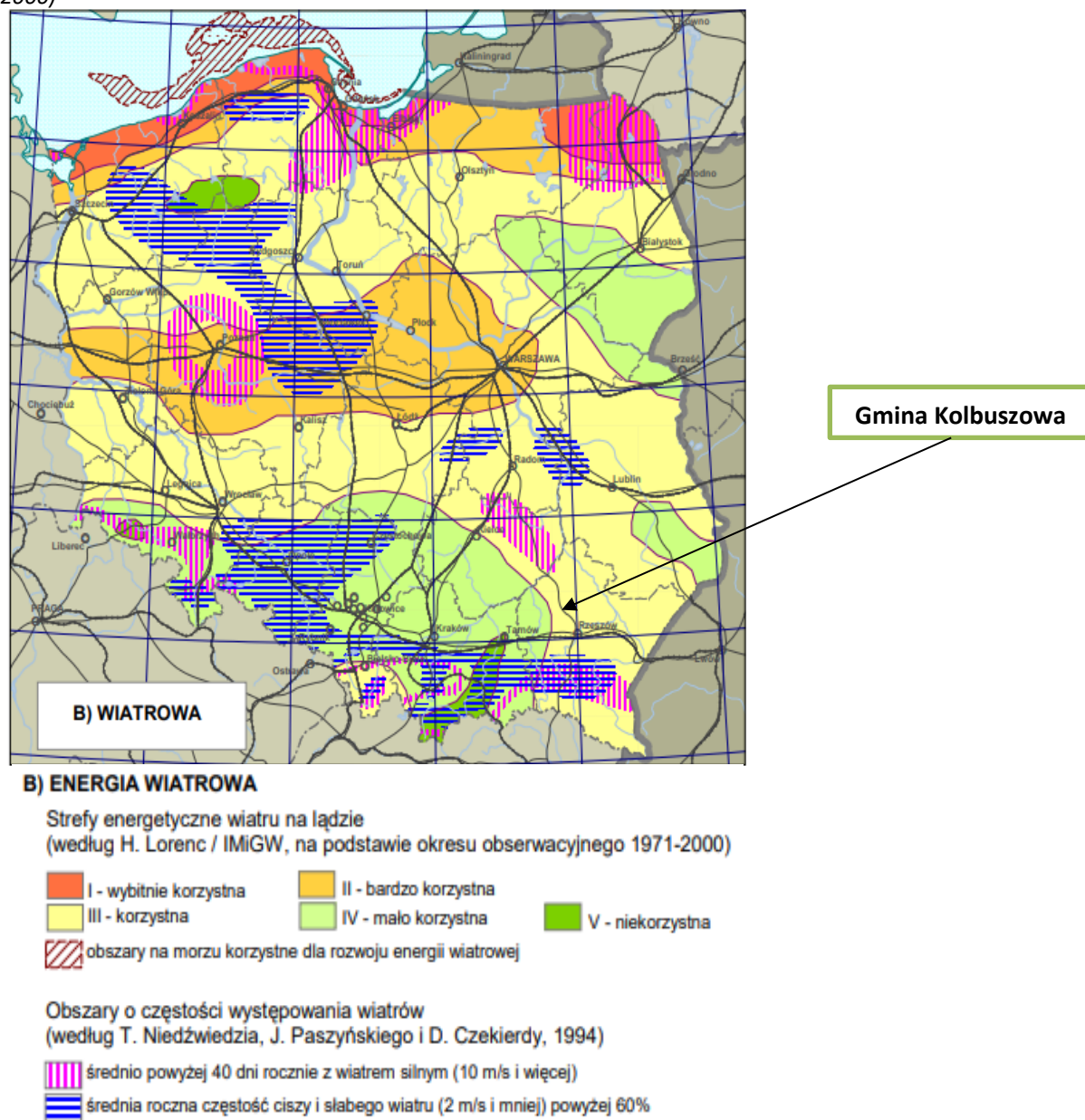
Rysunek 7. Strefy energetyczne wiatru na lądzie (według H. Lorenc/IMI GW, na podstawie okresu obserwacyjnego 1971-2000)
